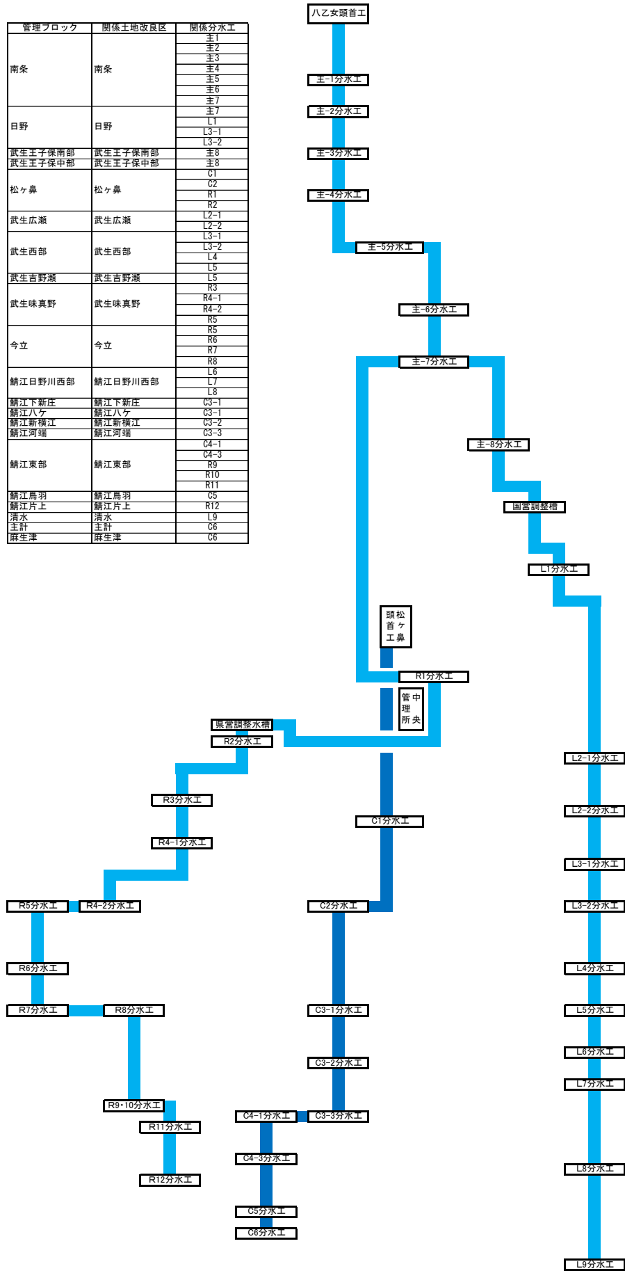
日野川用水土地改良区 管理ブロックおよび配水系統図
